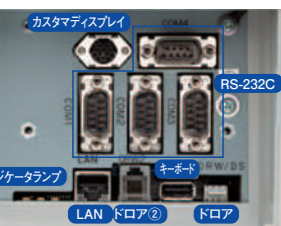
各種インターフェース(背面)
